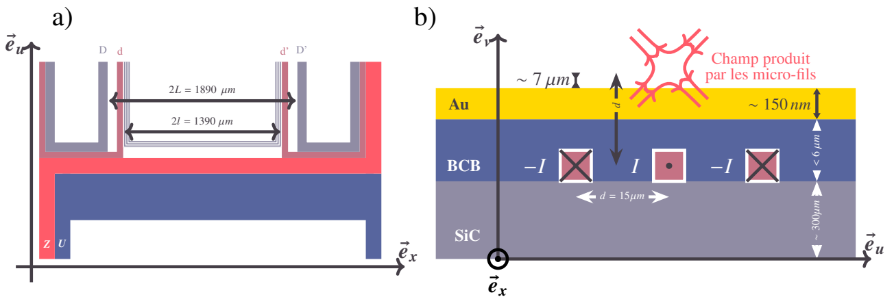
FIGURE 5.2 – a) Zoom sur la zone d'intérêt. Les fils U (bleu) et Z (rouge vif) créent des pièges magnétiques intermédiaires, les trois micro-fils gris forment le guide longitudinal, et les fils d/d' (marron) et D/D' (gris) assurent le confinement longitudinal. b) Schéma des différentes couches constituant la puce atomique.
